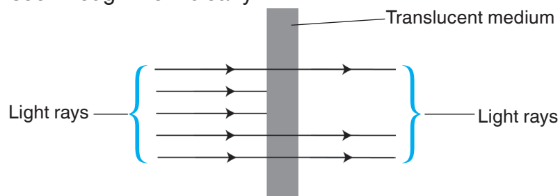
Fig. 14.2: Translucent medium.
