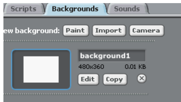
Fig. 7.19: Background menu.
