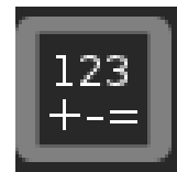
Fig. 7.4: Number palette.
