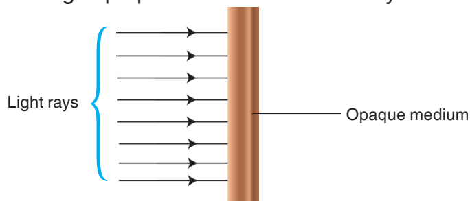
Fig. 14.3: Opaque medium.
