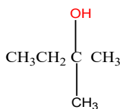
2Methylbutan-2-ol 2Methyl-2-butanol
