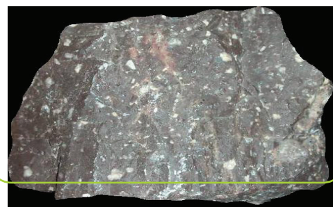
Lamprophyre.
