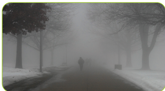
Fig 8.25 Fog.
