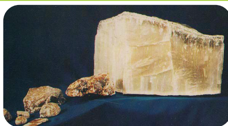
Trona.
